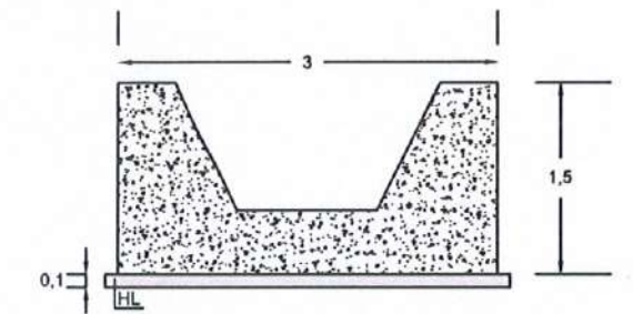
SECCIÓN D-D':CUNETA 2-POZO4
