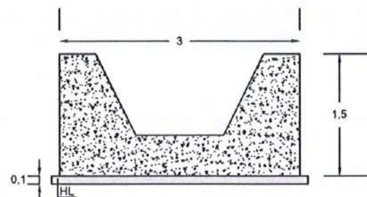
SECCIÓN B-B': CUNETA 2-POZO 3
