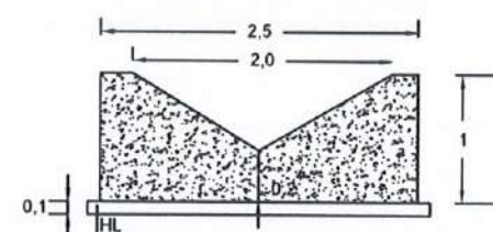
SECCIÓN C-C': CUNETAS 1-POZO2
