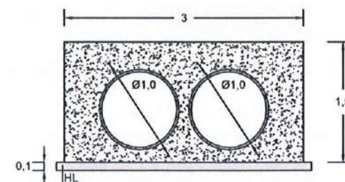
SECCIÓN E-E': POZO3- OF1
