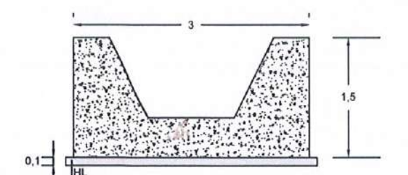
SECCIÓN F-F':CUNETA 2-POZO4
