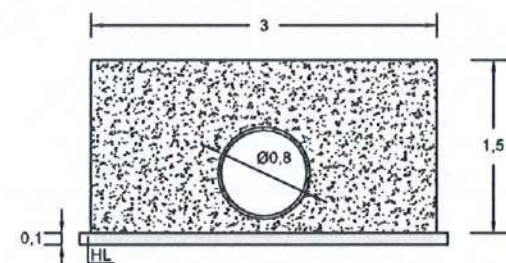
SECCIÓN C-C': POZO3-OF3
