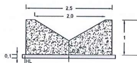
SECCIÓN B-B': CUNETAS 1-POZO 1
