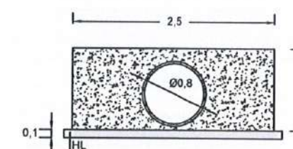
SECCIÓN D-D': CUNETAS 1-OF3
